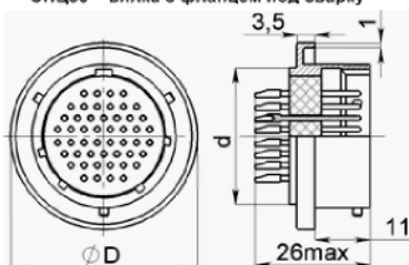
СНЦ30 – вилка с фланцем под сварку
