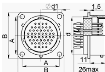
СНЦ31 – вилка с фланцем под винты
